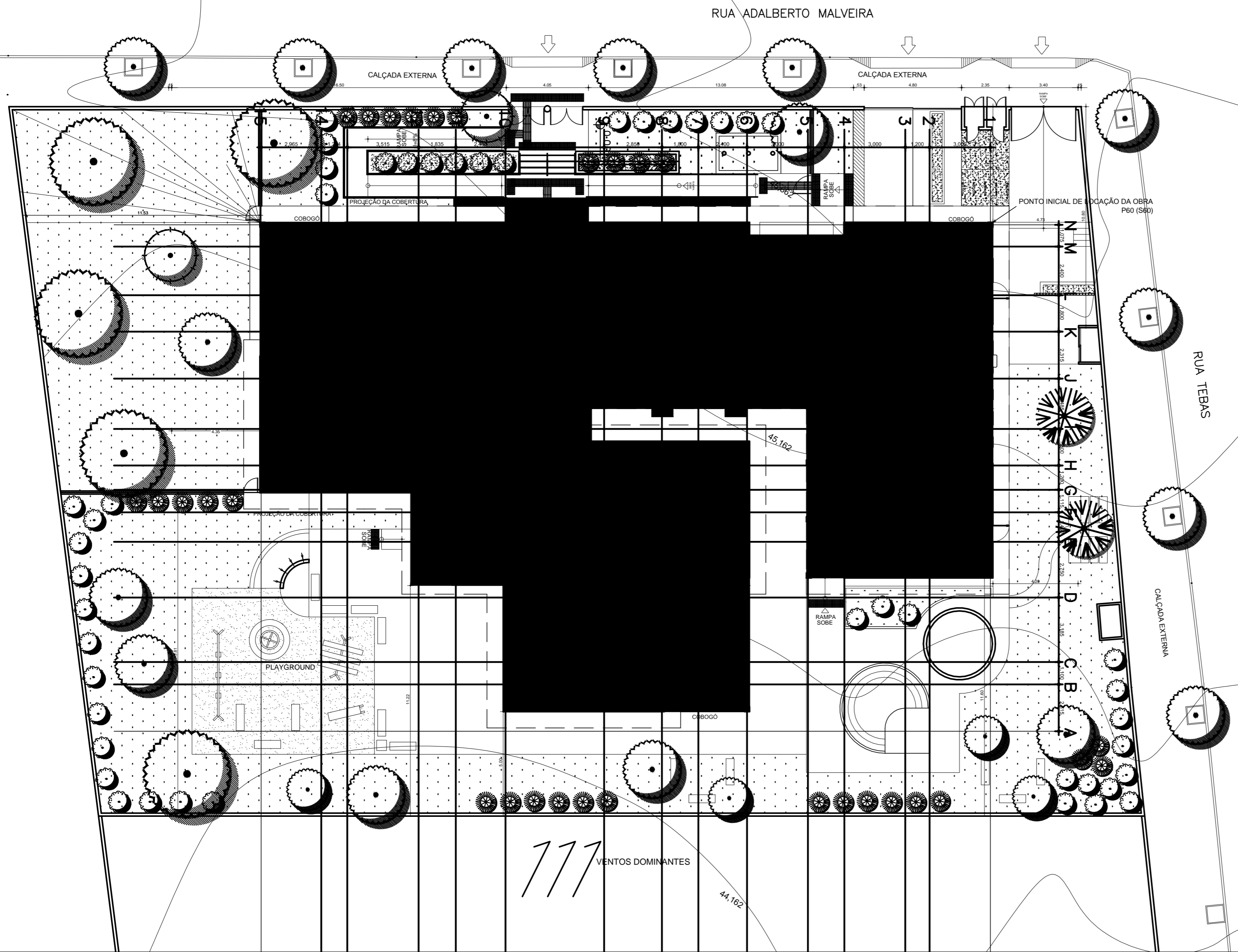
1 PLANTA DE LOCAÇÃO DOS PILARES ESC.: 1:150
